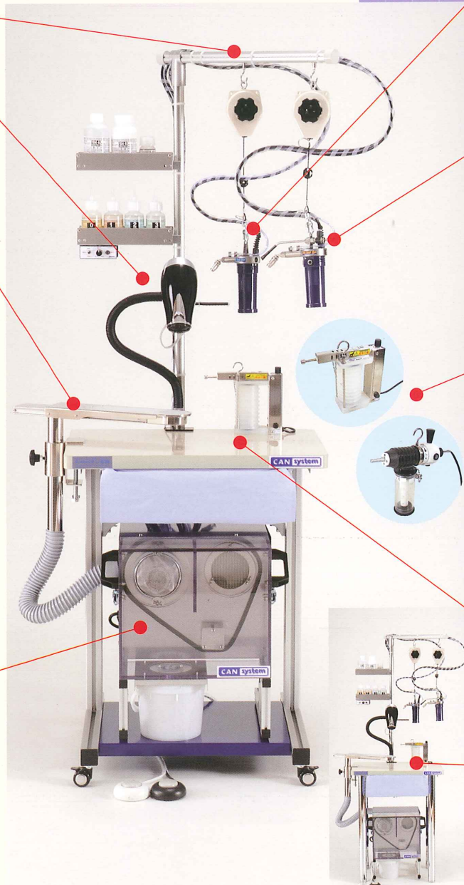
作業テーブル(移動型)(400×600)セット例
