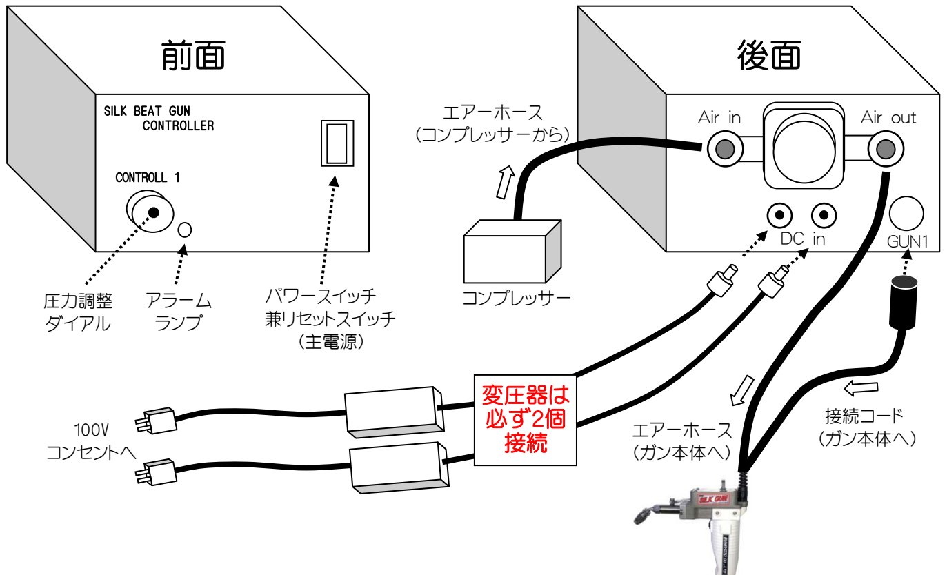
【電源BOX】 (図5) (Type/201-S II)
